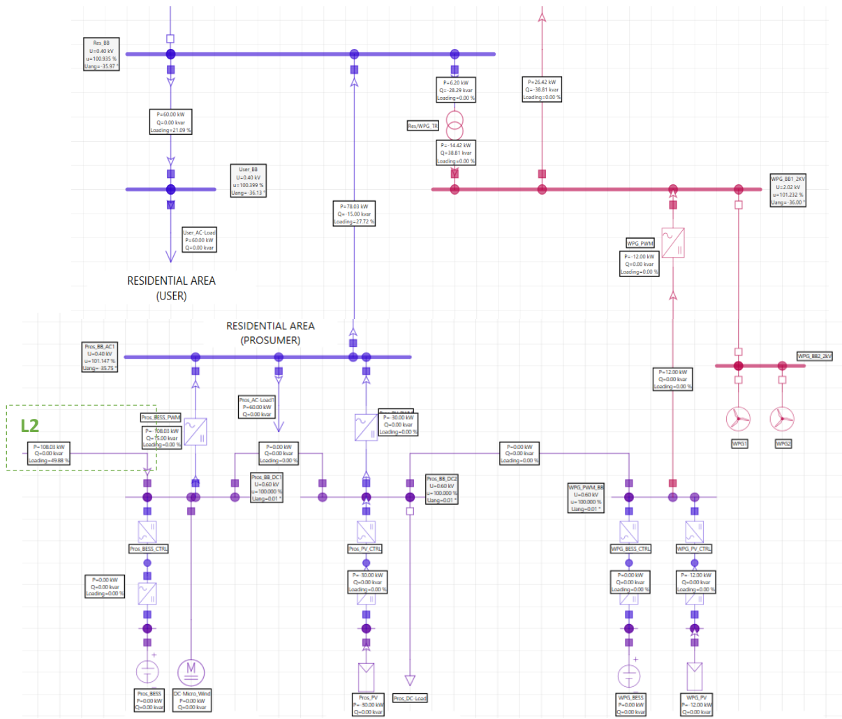
Figura 49. Sezione residenziale con linea di back-up chiusa, soccorso da parte delle risorse EVH.
