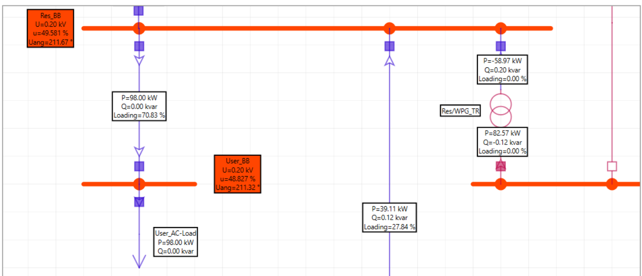
Figura 50. Sezione residenziale in condizione di islanding - Stato CA3-2020 (simulazione 1).
