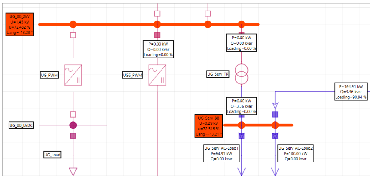
Figura 22. load flow in emergenza CA1-2020, simulazione 2.
