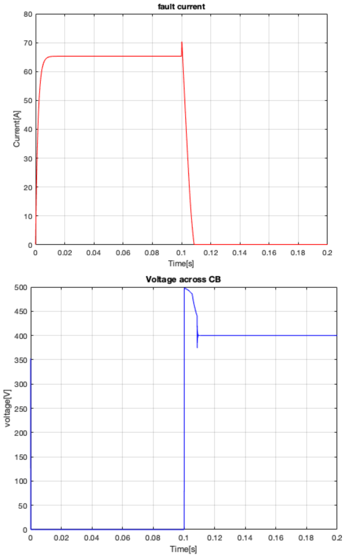
Figura 2.5: Comportamento di MOV SSCB in condizioni di guasto
