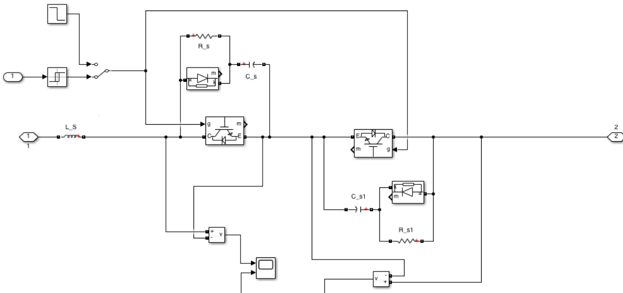
Figura 2.15: Configurazione RCD SSCB simulata nella rete DC simulata
