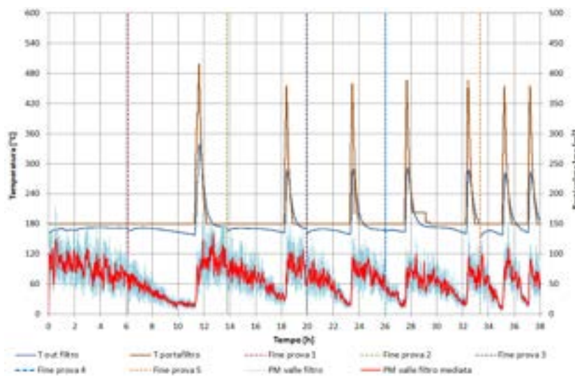
Figura 20. Confronto tra l’emissione di particolato a valle del filtro e le principali temperature misurate nelle prove sul secondo filtro a schiume ceramiche a media porosità
