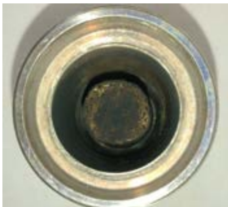
Figura 22. Vista dall'alto del secondo filtro a schiume ceramiche a media porosità nel suo alloggiamento al termine delle prove sperimentali
