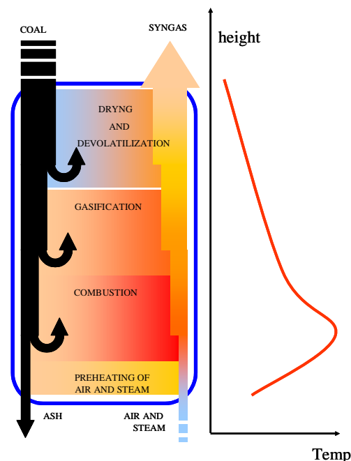
Figura 2. Profilo di temperatura e zone di reazione in un gassificatore updraft [4]
