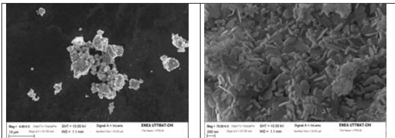
Figura 8 . Immagini SEM delle polveri di peroschite sintetizzate mediante ball milling (campione S2). La figura riporta immagini dello stesso campione a due diversi ingrandimenti.
