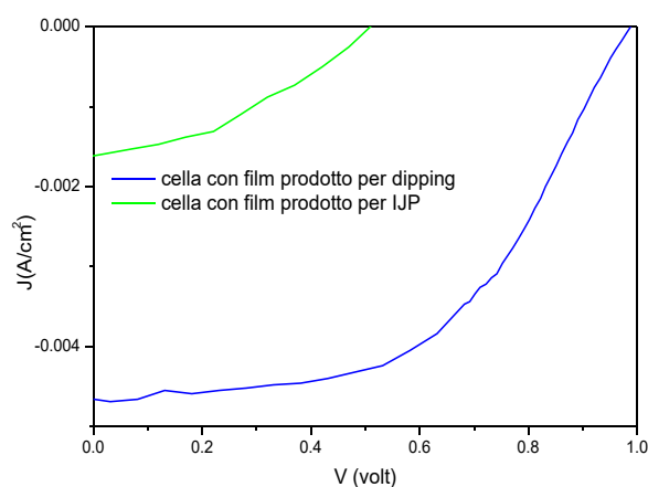
Figura 28. Curve J-V misurate sotto illuminazione a 100 \text{ mW/cm}^2 AM 1.5G nel caso di celle aventi struttura vetro/FTO/c-TiO 2 /m-TiO 2 /peroschite/HTM/oro prodotte con processo dual step mediante stampa IJP o dipping in una soluzione di ioduro di metilammonio.
