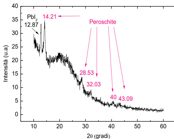
Figura 23. Spettro di diffrazione dei raggi X (Cu Kα) del campione S14 depositato su PEDOT:PSS.
