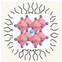
Figura 11. Schema di una peroschite funzionalizzata. Gli ioni di ottilammonio si dispongono sulla superficie del cristallo di peroschite aumentando la compatibilità del materiale con il solvente organico.
