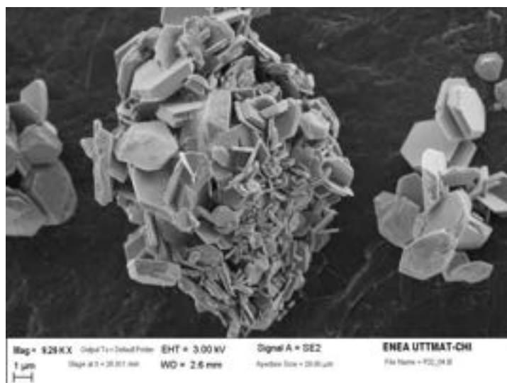
Figura 10. Immagine SEM del campione S8 sintetizzato in condizioni meno energetiche. La polvere è costituita da cristalli di peroschite dalla forma di piattelli esagonali assemblati in agglomerati di diversi micron.
