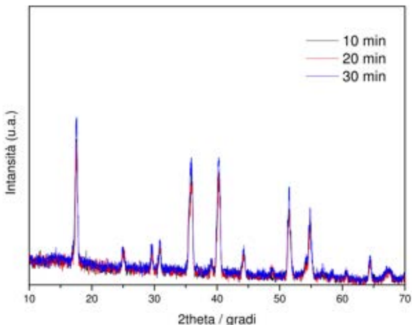
Figura 7. Spettri di diffrazione (Radiazione FeKα) delle polveri del campione S3 macinate per tempi crescenti (10, 20, 30 minuti). Tutti i picchi appartengono alla peroschite nella sua struttura tetragonale.
