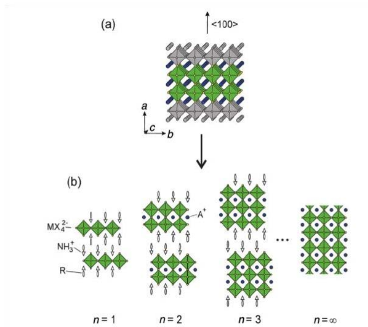
Figura 13. (a) Struttura della peroschite generica APbX_3 (nel presente lavoro A=CH_3NH_3^+ , X=I ) orientata lungo la direzione \langle 100 \rangle . I pallini blu corrispondono al catione organico metilammonio. Le strutture ottaedriche sono relative al metallo (Pb) circondato dall'alogenuro (I). (b) Famiglia di composti "intergrowth" dalla struttura bidimensionale o lamellare che si ripete lungo l'asse c. Questa è formata dall'alternarsi di strati di peroschite tridimensionale APbX_3 e peroschite bidimensionali dalla formula generica (RNH_3)_2PbX_4 , in questo studio R=ottille .
