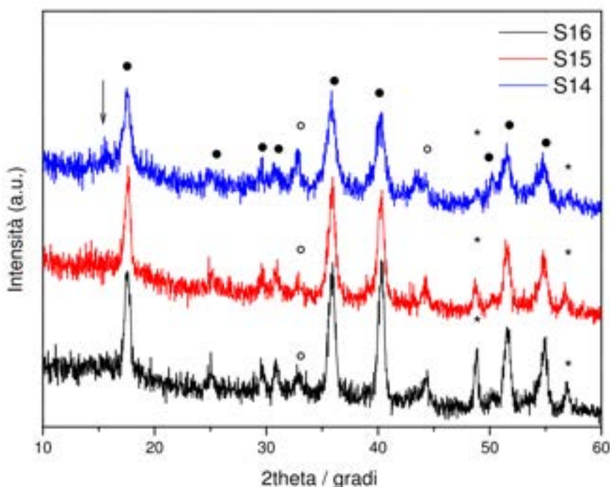
Figura 15. Spettri di diffrazione x (Radiazione \text{FeK}\alpha ) dei campioni S14, S15 e S16. In tutti e tre gli spettri, la peroschite \text{CH}_3\text{NH}_3\text{PbI}_3 è ben evidente e rappresenta la fase principale. Nello spettro del campione S14 compare una nuova fase indicata con una freccia. Tale picco è ascrivibile alla fase bidimensionale. (*) Al (portacampione); (°) \text{PbI}_2 .
