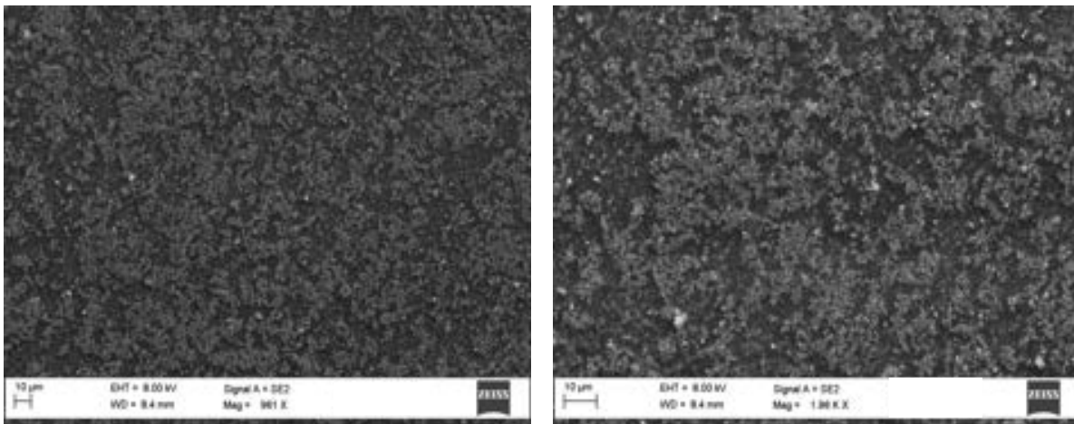
Figura 21. Immagini SEM della superficie di un film di peroschite S14 stampato su PEDOT:PSS.
