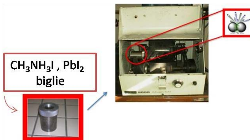
Figura 1. Rappresentazione schematica della meccanosintesi di polveri di CH_3NH_3PbI_3 in un mulino. La giara è caricata con le polveri dei precursori ( PbI_2 e MAI) e con delle biglie. Variando la massa e il numero di biglie è possibile modulare la natura del prodotto finale.
