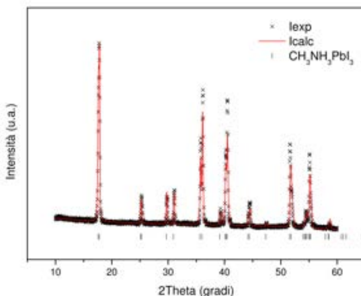
Figura 2 Analisi Rietveld di una polvere di peroschite sintetizzata mediante meccanochimica. La fase utilizzata ha gruppo spaziale I4cm . Parametri di cella raffinati: a=b=8.859\text{\AA} , c=12.613\text{\AA} , dimensione dei cristalliti 240\text{nm} , Rwp=0.17 . Radiazione \text{FeK}\alpha . Le linee verticali indicano le posizioni dei picchi.
