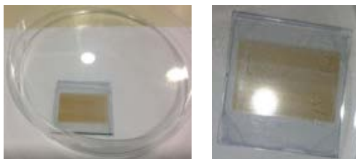
Figura 19. Immagini fotografiche di un film di peroschite ottenuto stampando su PEDOT:PSS un inchiostro a base di S14 in CB (3mg/mL).
