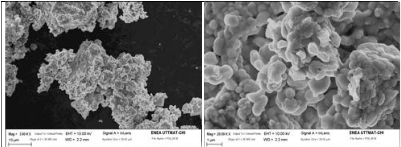
Figura 9 Immagini SEM delle polveri di peroschite sintetizzate mediante ball milling nelle stesse condizioni di S2 a partire da PbI_2 macinato. La figura riporta immagini dello stesso campione a due diversi ingrandimenti.
