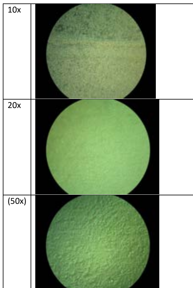
Figura 20. Immagini al microscopio ottico (prodotte a diverso ingrandimento) della superficie di un film di peroschite S14 stampato su PEDOT:PSS.
