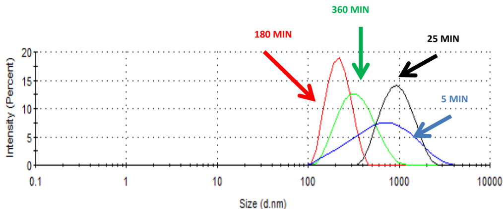
Figura 18. Curve di distribuzione delle dimensioni idrodinamiche delle particelle di peroschite S14 disperse in CB ottenute dopo diversi tempi di trattamento in bagno ultrasonico.
