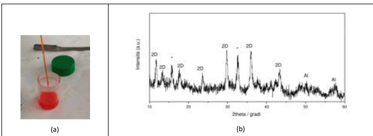
Figura 14. In (a) è riportata la foto di una dispersione di peroschite mista organica-inorganica bidimensionale (OA)_2PbI_4 in clorobenzene. In (b) lo spettro di diffrazione della polvere (radiazione FeK\alpha ). I principali picchi della fase bidimensionale sono indicati con "2D". "Al" indica i picchi relativi al portacampione di alluminio e "*" dello ioduro di piombo non reagito.
