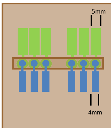
Figura 3. Schema dei dispositivi cella con struttura vetro/ITO (verde)/PEDOT:PSS/peroschite (striscia rettangolare marrone)/PCBM (quadrato esterno marrone)/Al (blu).
