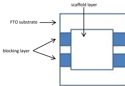
Figura 4: Schema del substrato utilizzato per la deposizione dello ioduro di metilammonio (sintesi in due fasi della peroschite): strato blocking (c-TiO 2 ) su vetro/FTO, ricoperto da uno strato scaffold (m-TiO 2 ). La geometria del substrato è tale da realizzare quattro celle da 0.1cm 2 di area.
