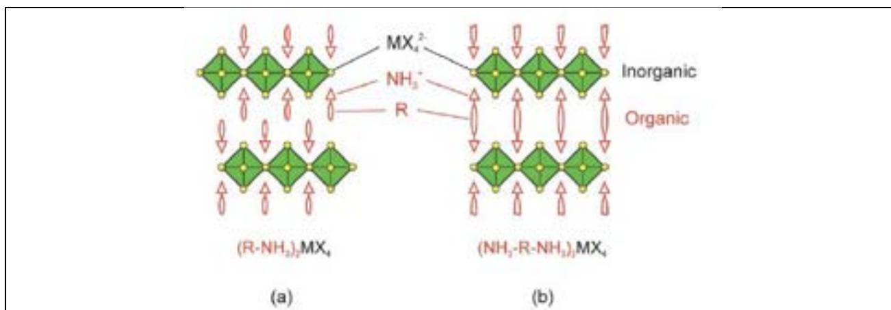
Figura 12. Descrizione schematica di uno strato di peroschite lamellare bidimensionale (2D) orientata lungo la direzione (100). In (a) è utilizzato un monocatione ammonio organico ( \text{RNH}_3^+ ), scelta adottata in questa sperimentazione. In (b) si è fatto uso di cationi di-ammonio organici ( ^+\text{NH}_3\text{RNH}_3^+ ).
