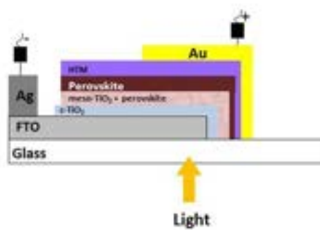
Figura 6. Schema dell'architettura utilizzata nella realizzazione della cella a base di peroschite non funzionalizzata: vetro/FTO/c-TiO 2 /m-TiO 2 /peroschite/HTM/oro.
