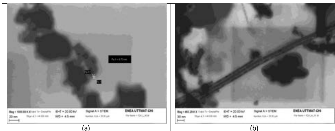
Figura 17. Immagini STEM di materiali sintetizzati aggiungendo OAI all’ambiente di reazione. In (a) sono visibili cristalli di peroschite funzionalizzata con catena di ottillammonio (campione S16). La fase organica è visibile come alone chiaro intorno al cristallo ad ha uno spessore intorno ai 5nm. In (b) un’immagine del campione S14 in cui accanto alla peroschite funzionalizzata è ben distinguibile un cristallo lamellare di peroschite 2D. Lo strato di peroschite mista organica-inorganica (scuro) è intervallato da materiale organico (più chiaro).
