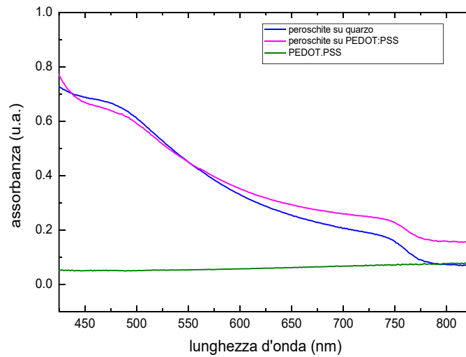
Figura 24. Spettro di assorbimento di film di peroschite prodotti per stampa su substrati di quarzo con e senza uno strato intermedio a base di PEDOT:PSS.
