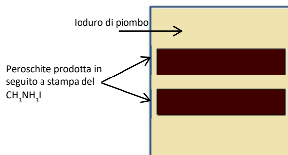
Figura 5. Schema delle strisce di peroschite ottenute dalla reazione dello ioduro di metilammonio sul film di ioduro di piombo.
