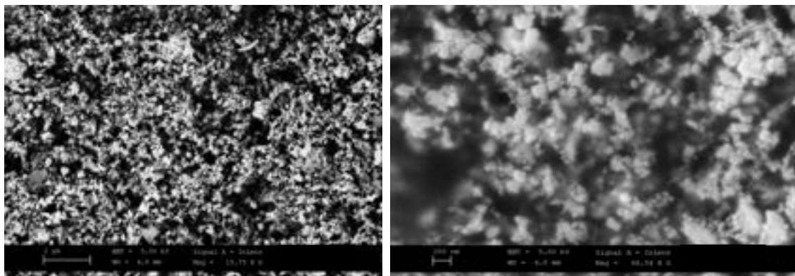
Figura 27. Immagini SEM (a diverso ingrandimento) del film di perovskite funzionalizzata prodotto per stampa e introdotto nella struttura della cella secondo lo schema di Figura 26.
