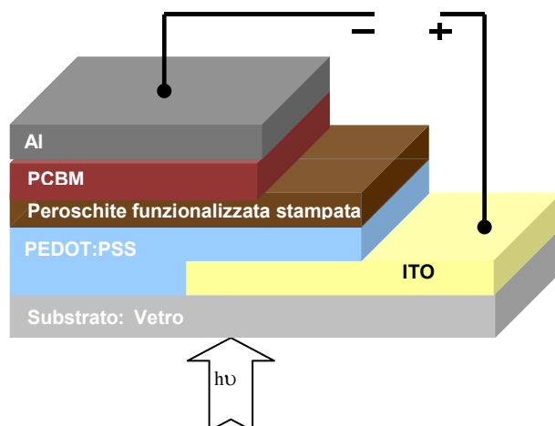
Figura 26. Schema dell'architettura della cella a base di perovskite funzionalizzata: vetro/ITO/PEDOT:PSS/perovskite/PCBM/Al.
