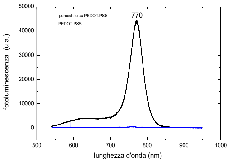
Figura 25. Spettri di fotoluminescenza (lunghezza d'onda di eccitazione 514nm) di un film di peroschite stampato su PEDOT: PSS (nero) e, per confronto, di solo PEDOT:PSS (blu).
