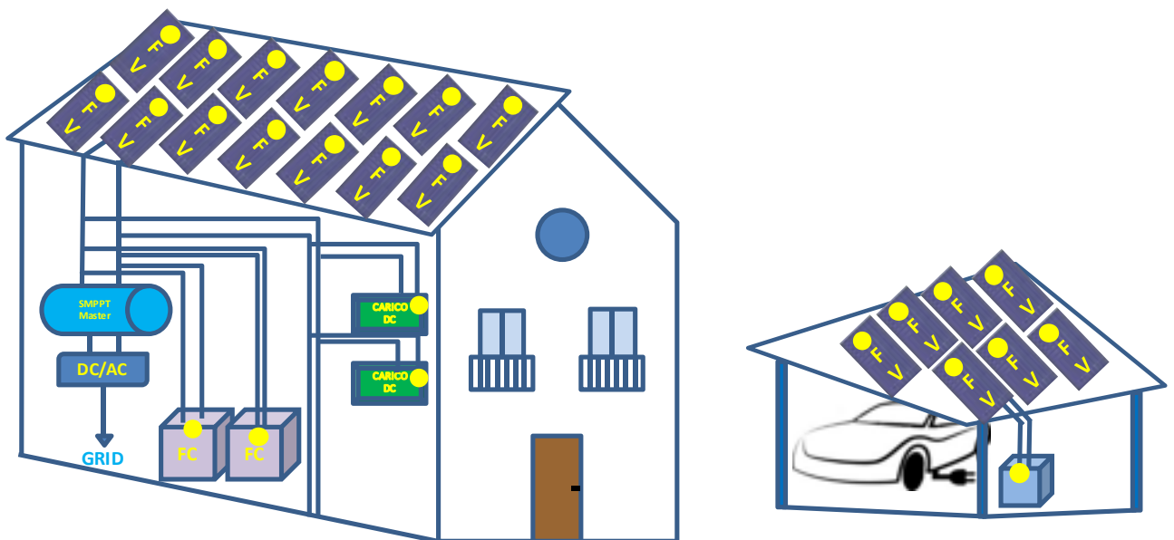
Figura 2. Architettura di convertitori SMPPT in una micro rete DC.
