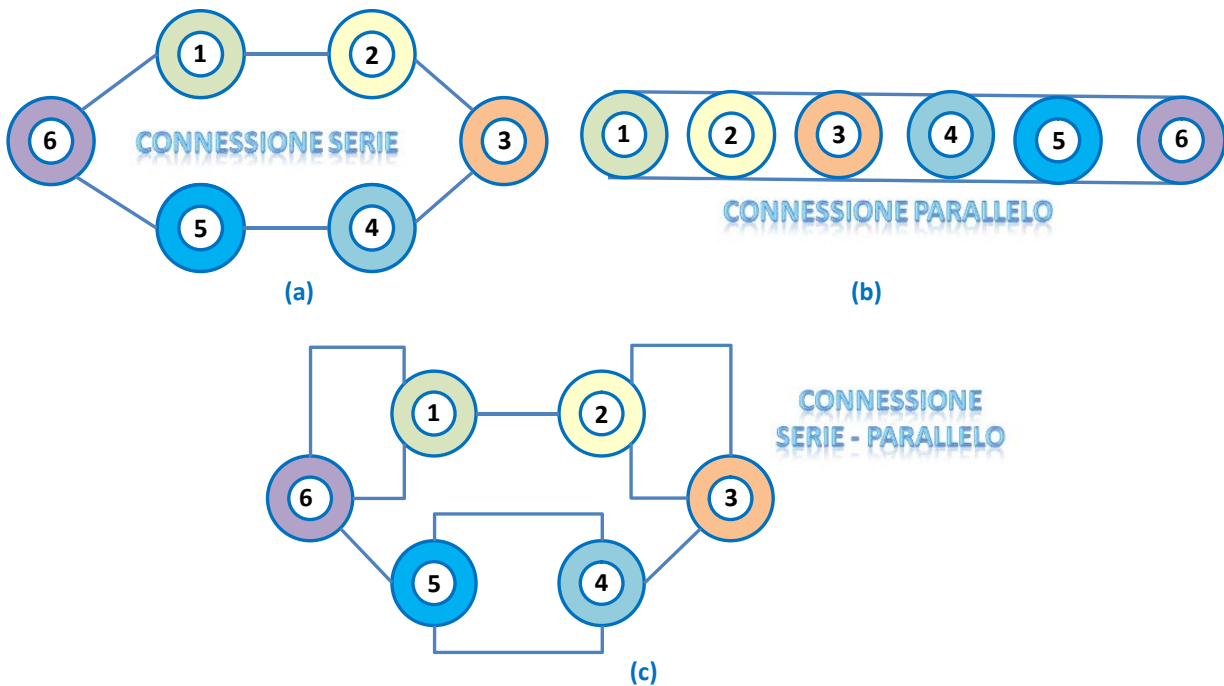
Figura 12. a. Connessione di tipo serie; b. Connessione di tipo parallelo; c. Connessione serie/parallelo.
