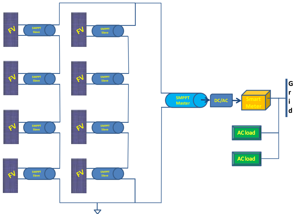
Figura 1. Architettura Master-Slave di convertitori SMPPT in un impianto fotovoltaico.
