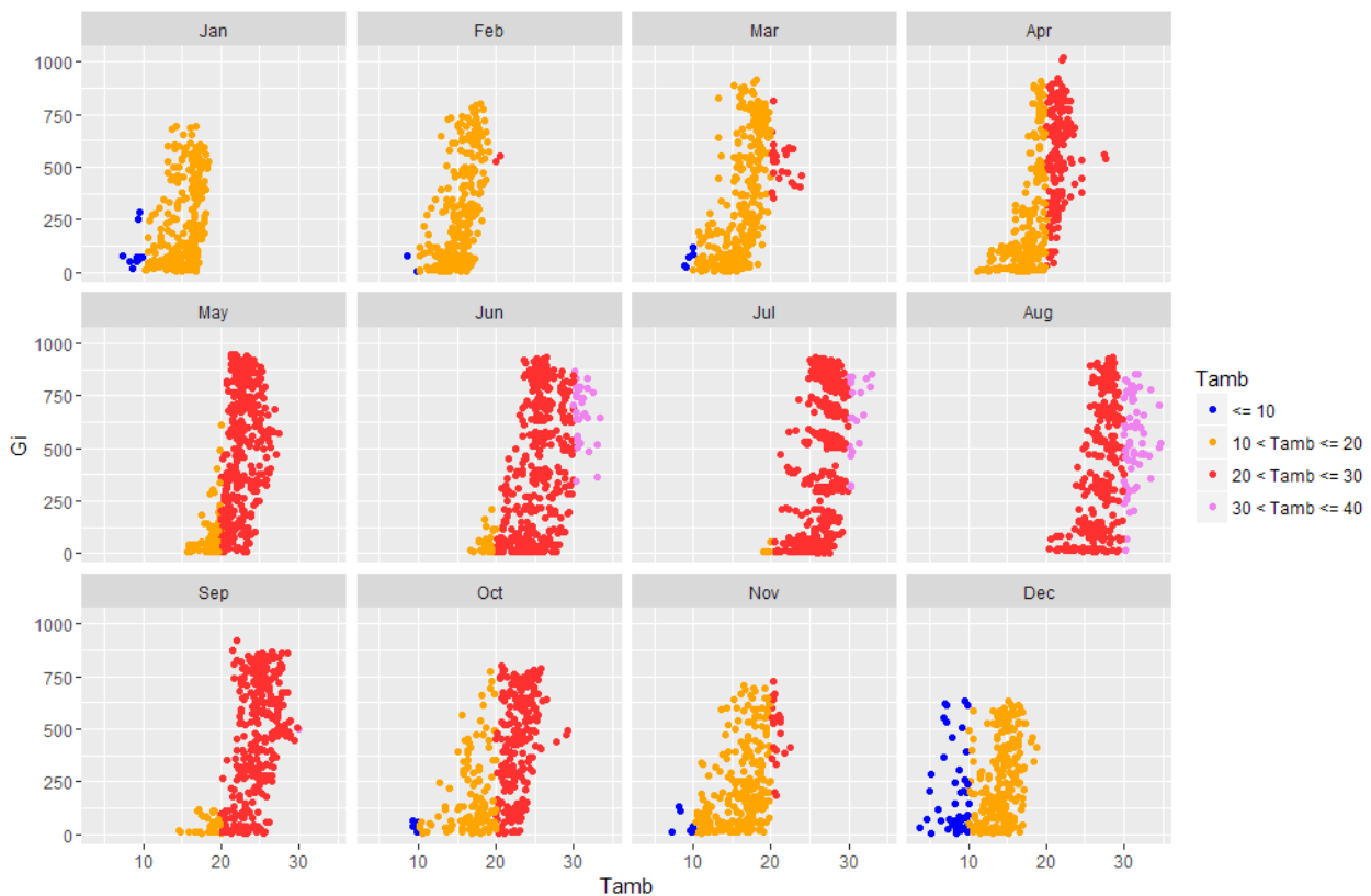
Figura 10. Distribuzione annuale temperatura ambiente e soleggiamento.
