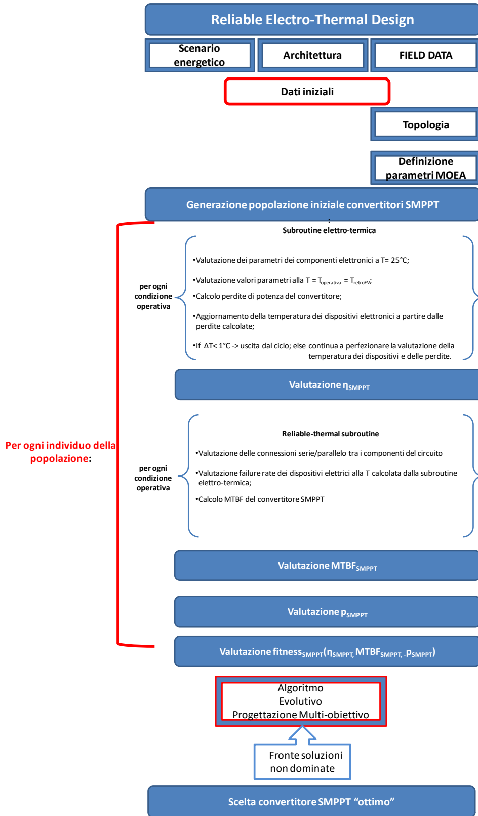
Figura 14. Schema sintetico del tool RET.
