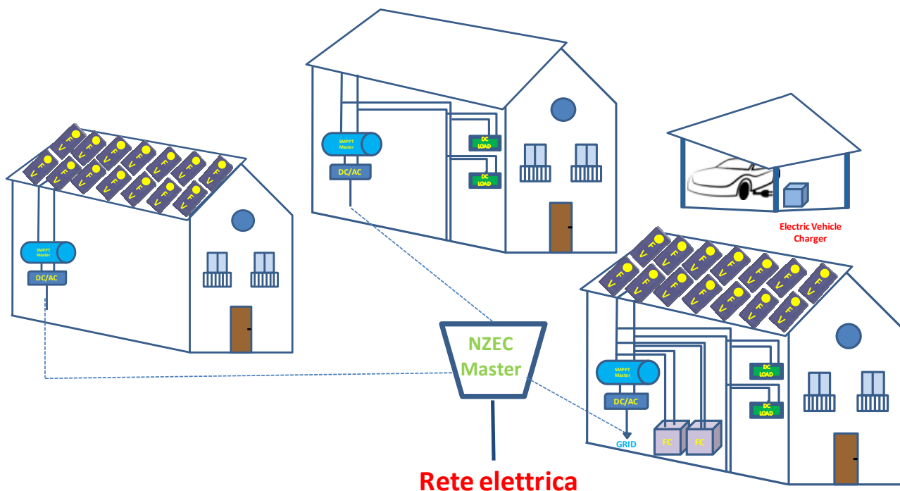
Figura 3. Architettura di convertitori SMPPT in un Net Zero Energy Cluster.
