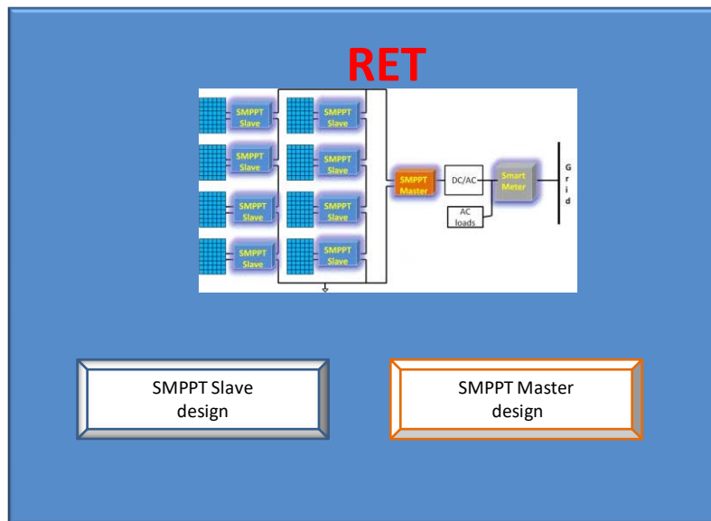
Figura 15. RET: interfaccia di progettazione per Master-Slave SMPPT.
