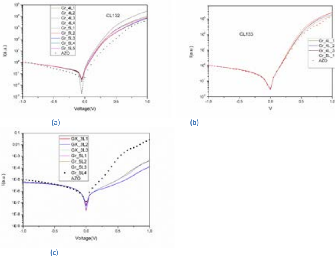
Figura 11. Caratteristiche corrente tensione (normalizzate per favorire il confronto) al buio delle celle del gruppo CL132 (a), CL133(b) e CL134). In ciascun grafico è riportato il confronto con il dispositivo avente l’elettrodo in AZO
