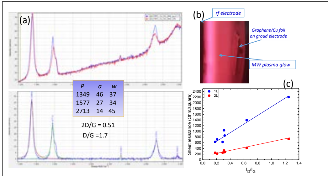
Figura 3. (a) Spettri Raman di grafene su rame dopo trattamento con plasma di azoto. Si evidenzia la presenza del picco D. (b) Foto del bagliore di plasma a radiofrequenza (13.56 MHz) durante il trattamento del grafene in condizioni di plasma modulato (MW). (c) Correlazione della sheet resistance e del rapporto picco D e picco G ( I_D/I_G ) per grafene monolayer e bilayer trasferiti su Corning glass e sottoposti a plasma di N_2 per diversi tempi di esposizione: un aumento del picco dei difetti corrisponde ad un aumento della sheet resistance.
