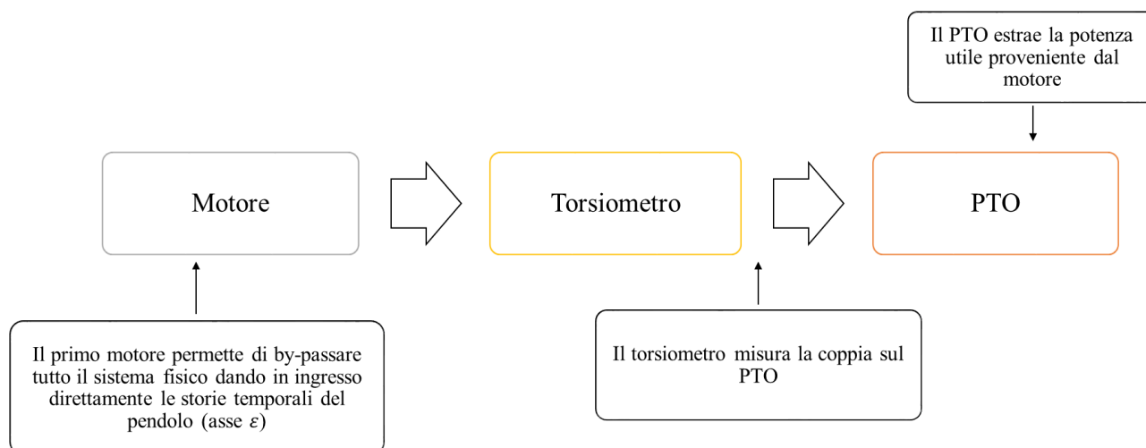
Figura 1: Schema concettuale banco prova.
