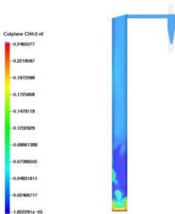
Figura 39. Frazione molare di CH 4 . Caso 3
