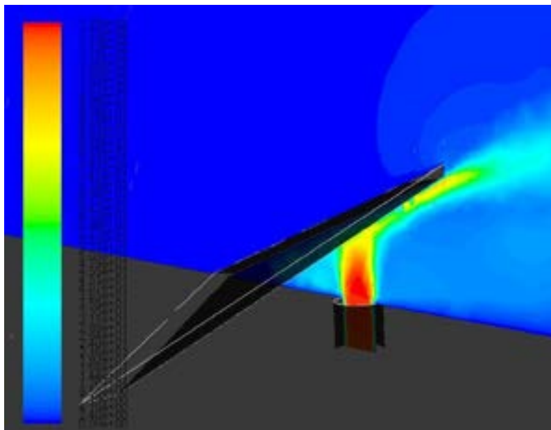
Figura 10. Mappa delle velocità (m/s) per l'iniettore
