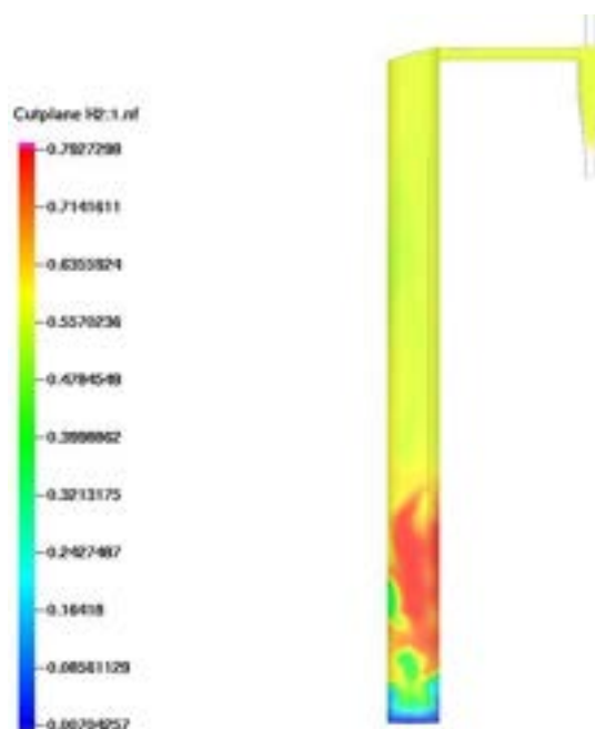
Figura 39. Frazione molare di H_2 . Caso 3
