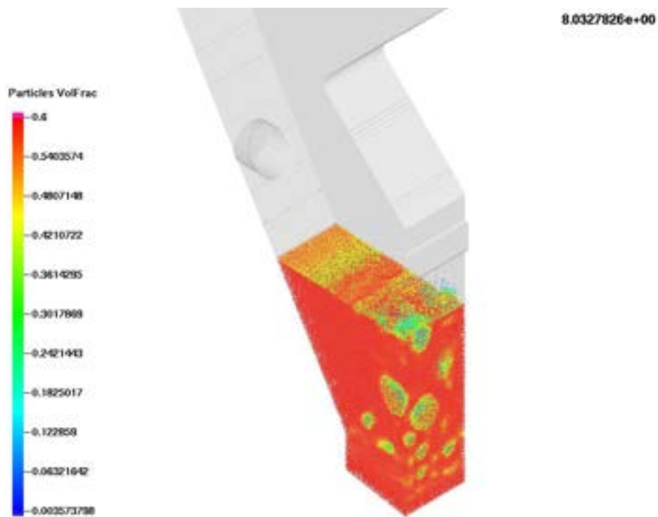
Figura 21. Caso (C3, P2)
