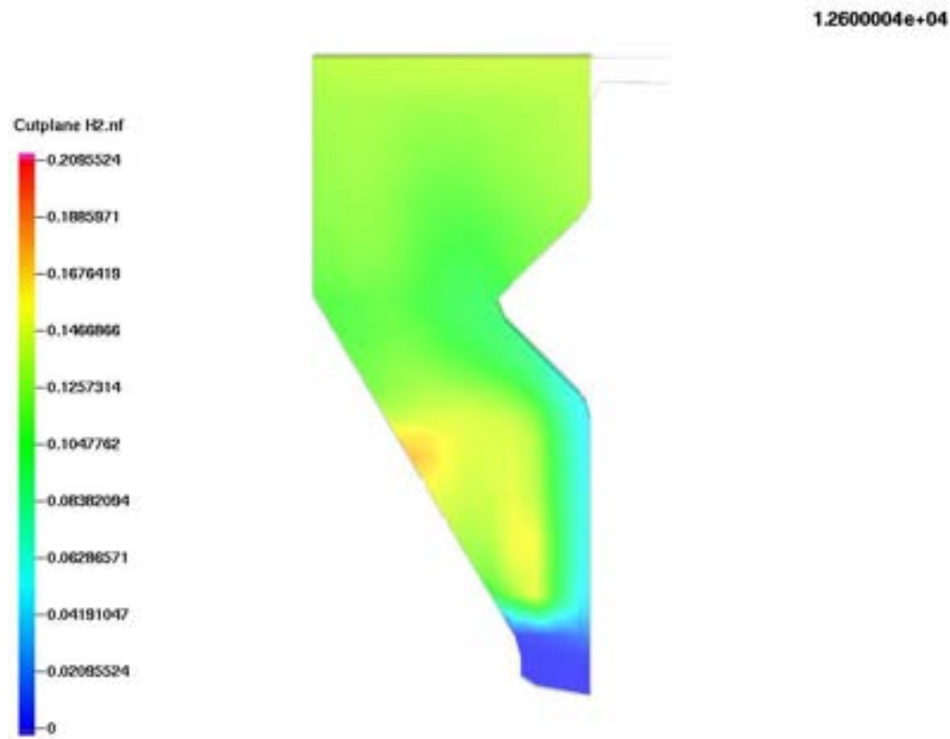
Figura 25. Frazione in volume di H 2
