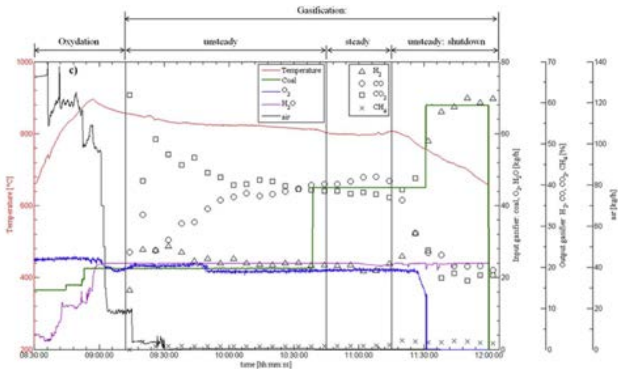
Figura 29. Risultati sperimentali della gassificazione
