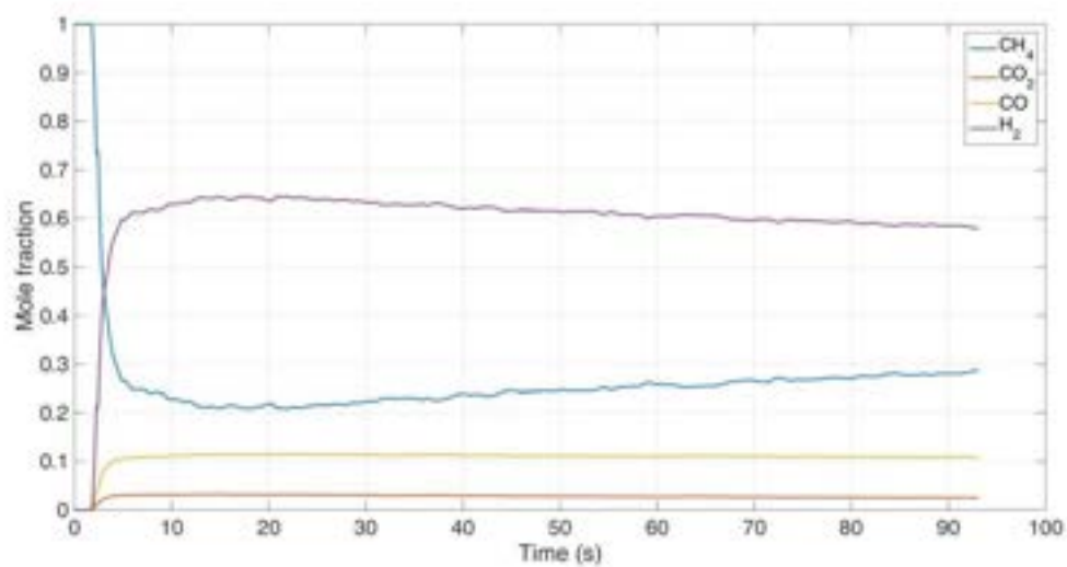
Figura 36. Frazione molare (su base secca) delle specie all'uscita. Caso 2
