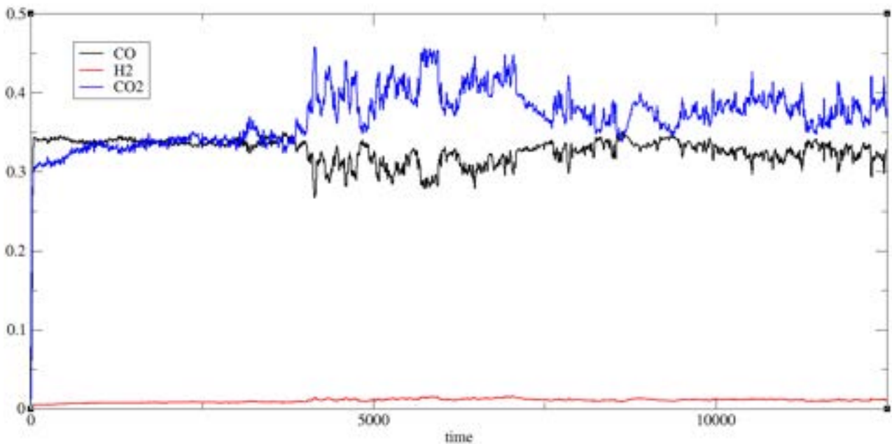
Figura 28. Andamento temporale di: CO, H 2 , CO 2
