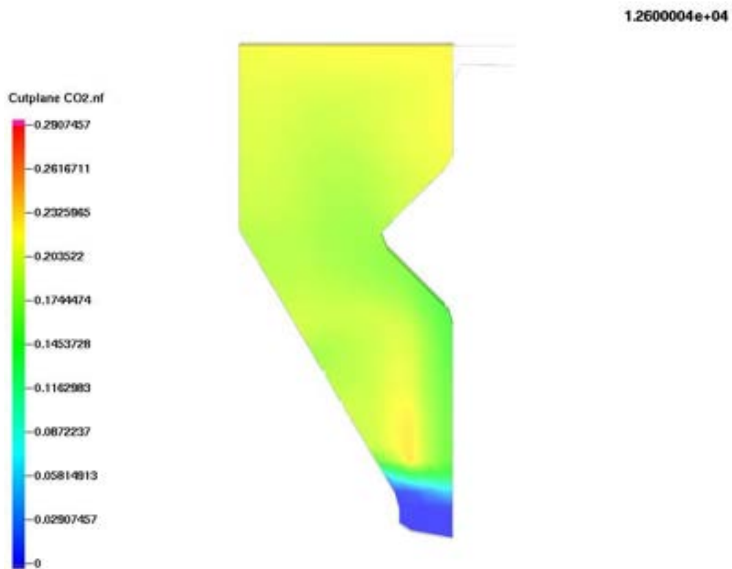
Figura 26. Frazione in volume di CO 2
