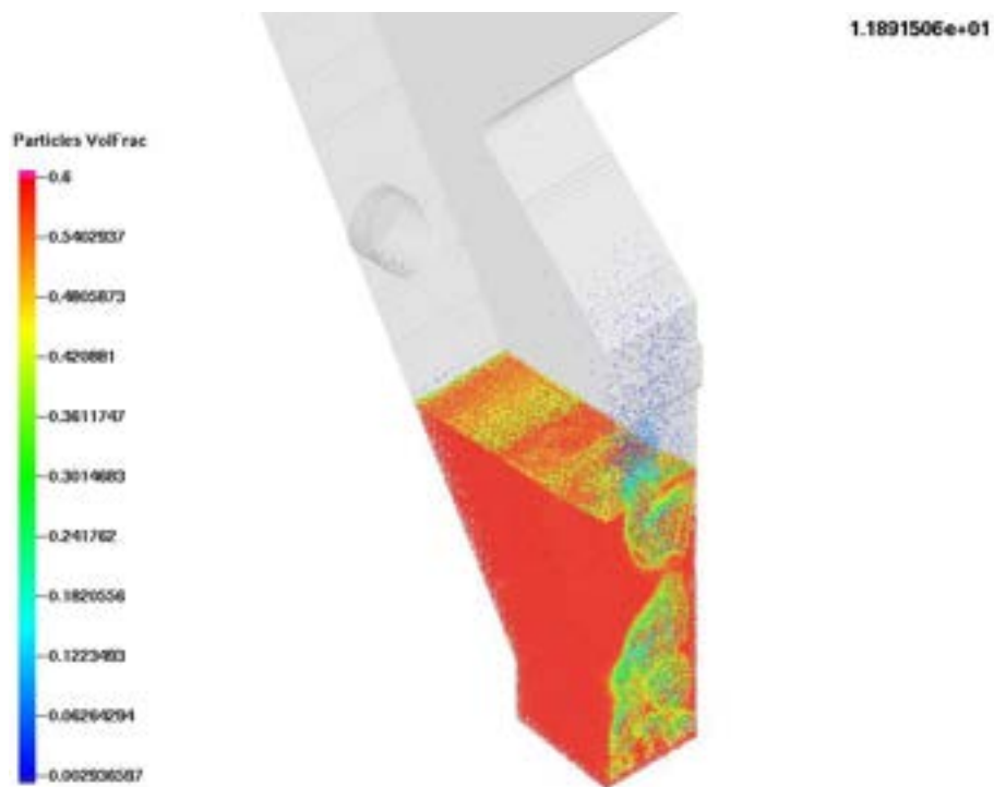
Figura 17. Caso (C1, P2)
