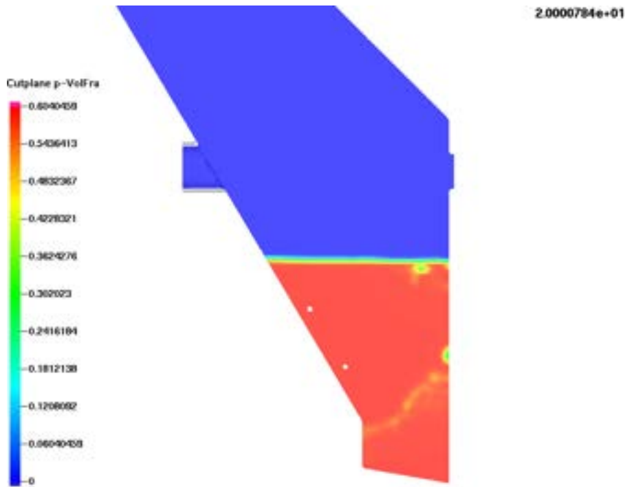
Figura 16. Caso (C3, P1) sezione
