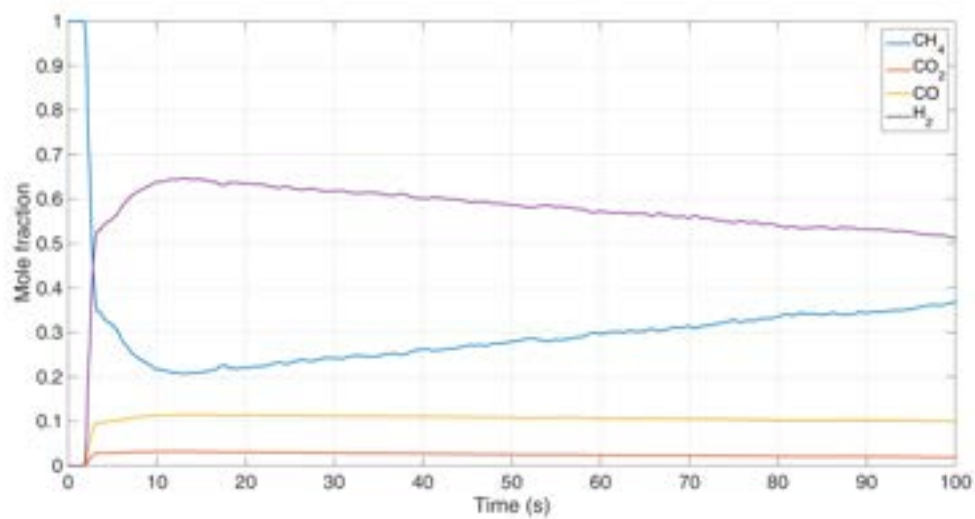
Figura 35. Frazione molare (su base secca) delle specie all'uscita. Caso 1
