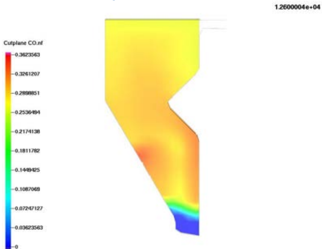
Figura 27. Frazione in volume di CO
