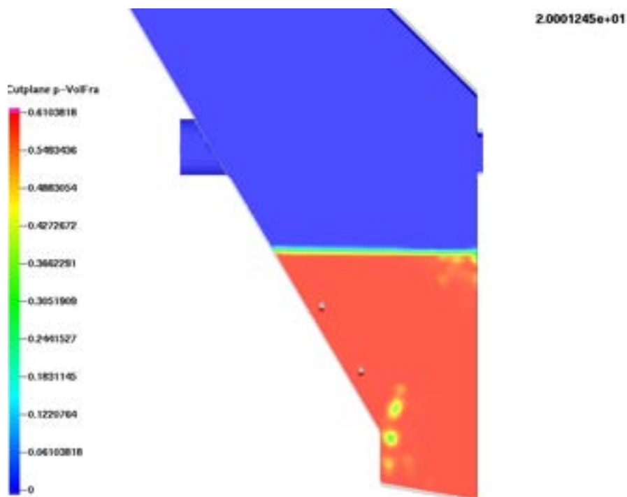
Figura 14. Caso (C2, P1) sezione
