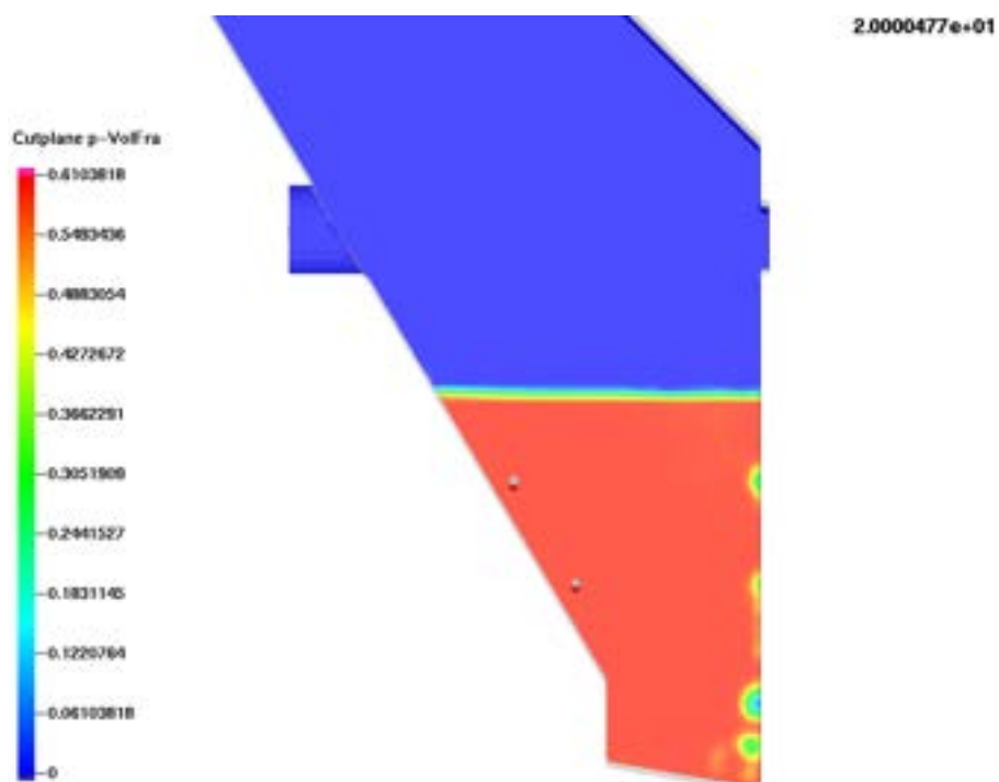
Figura 12. Caso (C1, P1) sezione
