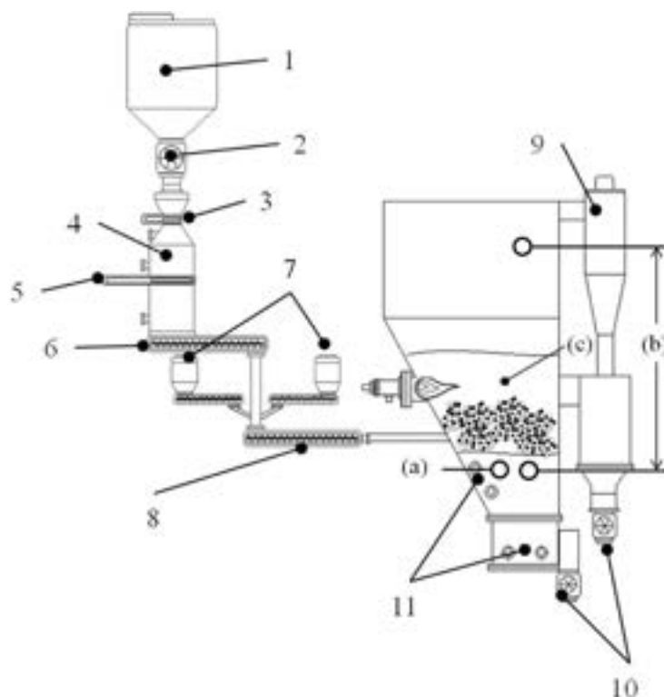
Figura 1. Schema del Gassificatore pilota
