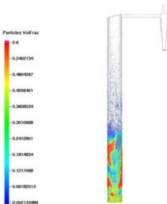
Figura 38. Frazione di volume delle particelle. Caso 3.
