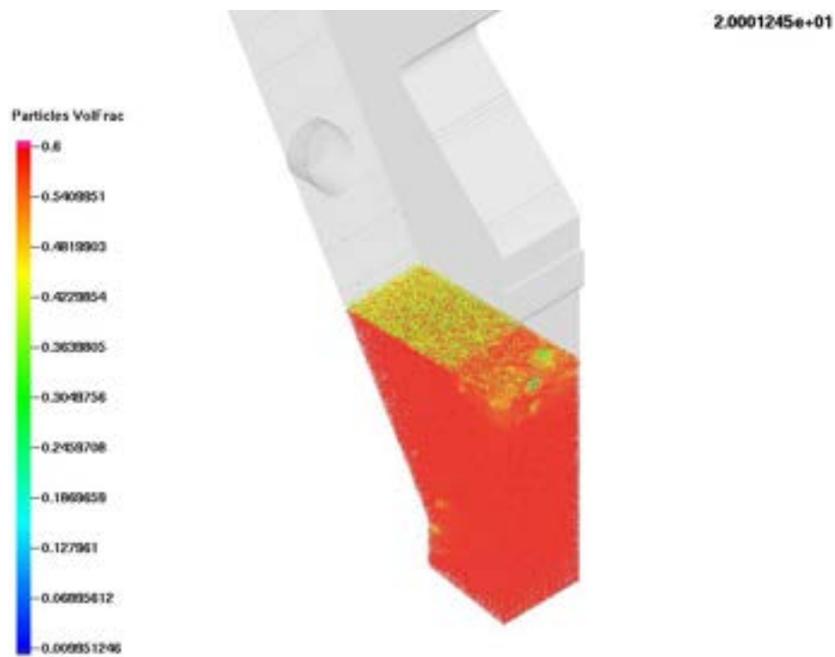
Figura 13. Caso (C2, P1)
