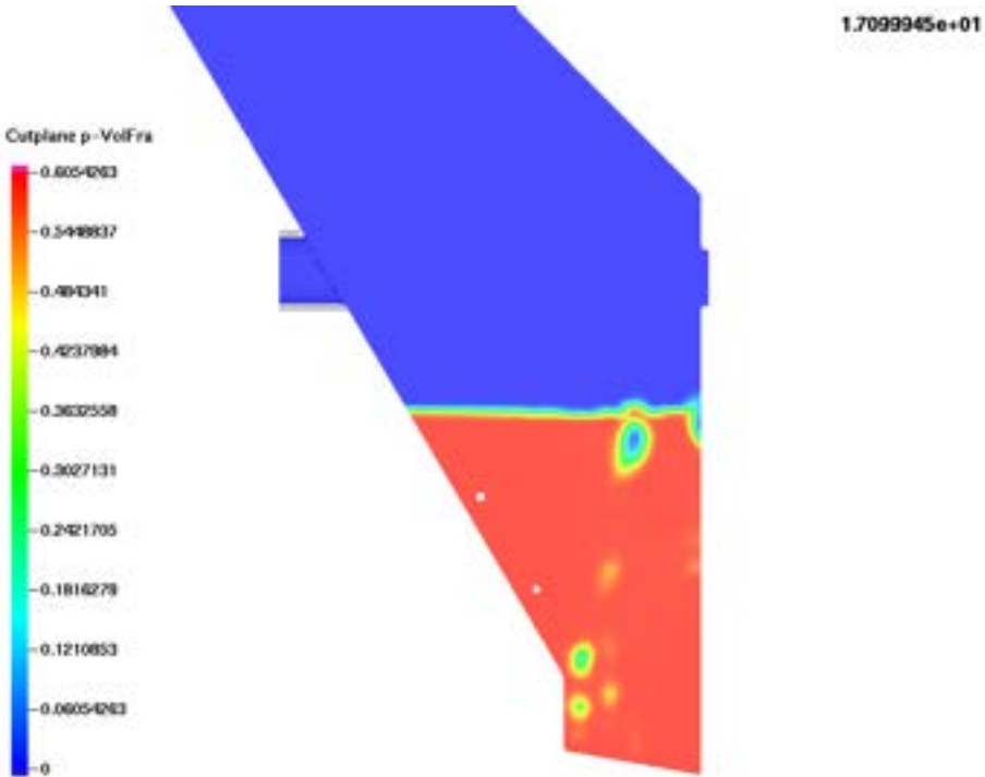
Figura 20. Caso (C2, P2) sezione
