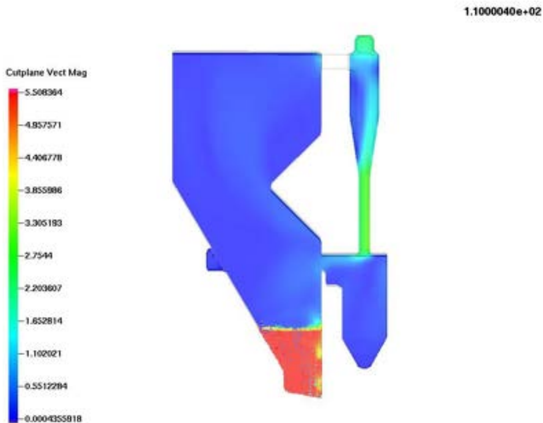
Figura 23. Campo di velocità (m/s)
