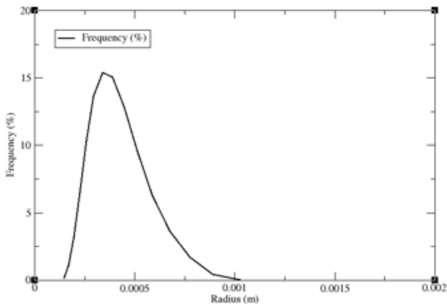
Figura 9. Distribuzione dei raggi delle particelle di olivina
