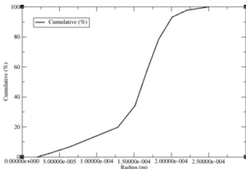
Figura 34. Distribuzione cumulativa delle particelle di dolomite
