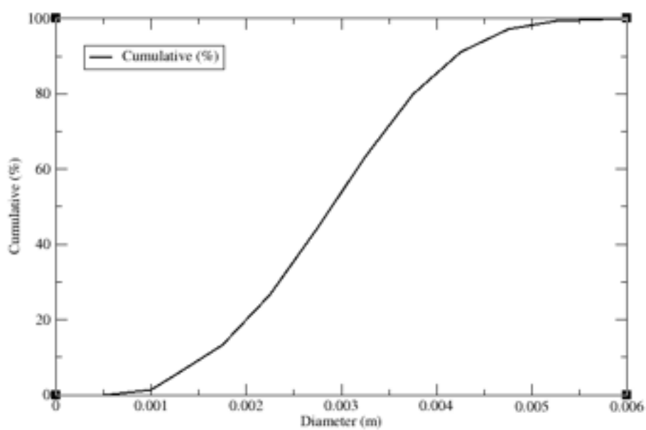
Figura 8. Distribuzione dei diametri delle particelle di carbone
