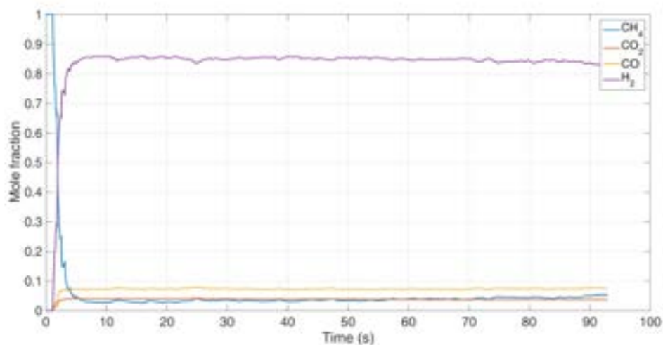
Figura 37. Frazione molare (su base secca) delle specie all'uscita. Caso 3
