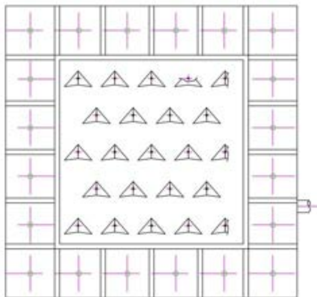
Figura 3. Distribuzione ugelli di alimentazione Gas di Fluidizzazione/Gassificazione
