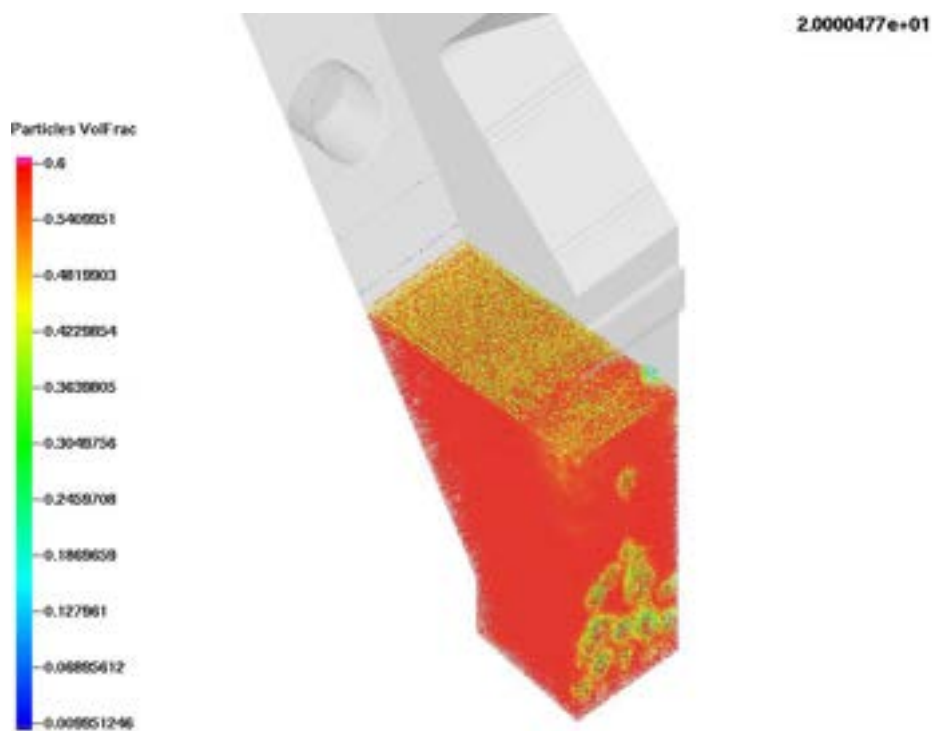
Figura 11. Caso (C1, P1)
