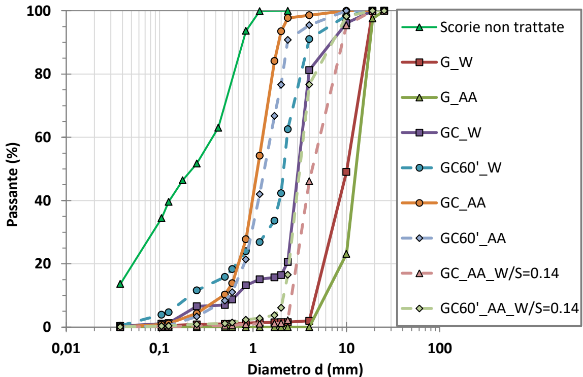
Figura 9 Curva di distribuzione granulometrica dei granuli ottenuti dopo i trattamenti testati (da Morone et al., 2016 [19])
