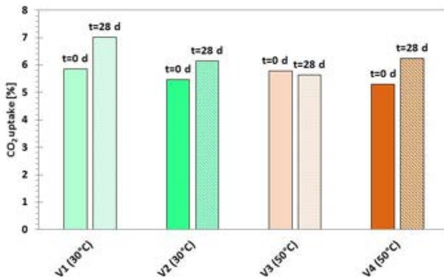
Figura 18 \text{CO}_2 uptake [%] dei granuli ottenuti a seguito dei test di granulazione-carbonatazione nel reattore a tamburo rotante, subito dopo la fine della prova (t=0 d) e dopo 28 giorni di curing (t=28 d) (da Librandi et al., 2016, [21])
