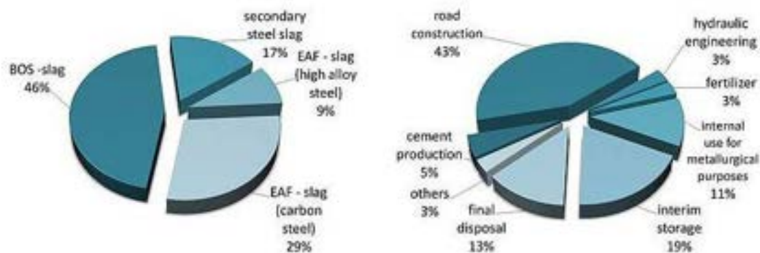
Figura 1 Produzione e riutilizzo di scorie di acciaieria [1]
