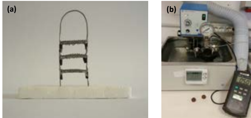
Figura 6 (a) Porta campioni in fil di ferro; (b) rettore in acciaio e bagno termostatico
