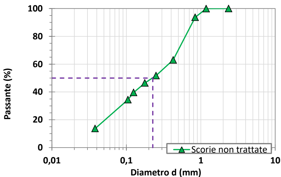
Figura 8. Curva granulometrica scorie BOF
