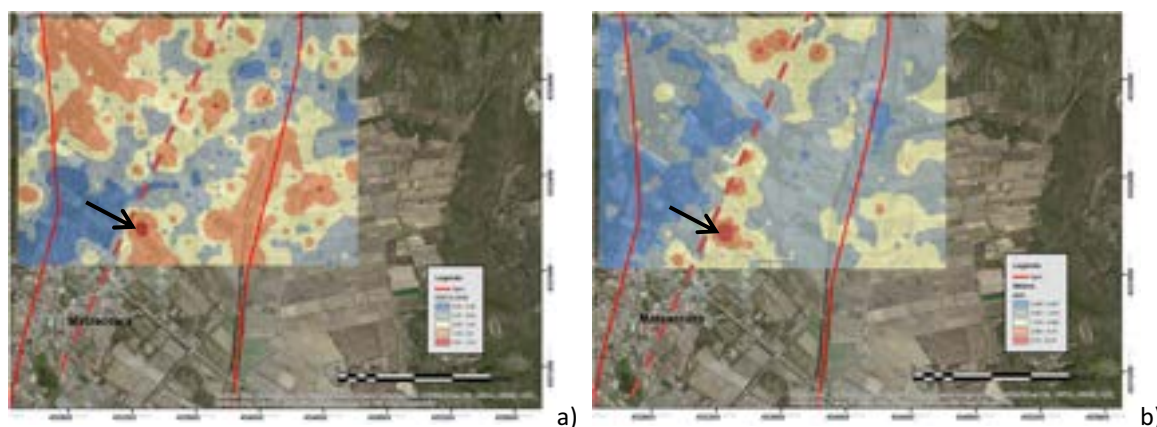
Figura 8. Concentrazioni di CO 2 (a) e CH 4 (b) misurate nel 2015 dal personale CERI-Sapienza (Bigi et al., 2015). Le frecce indicano l'area anomala che è stata ricampionata in questo lavoro per le analisi isotopiche.
