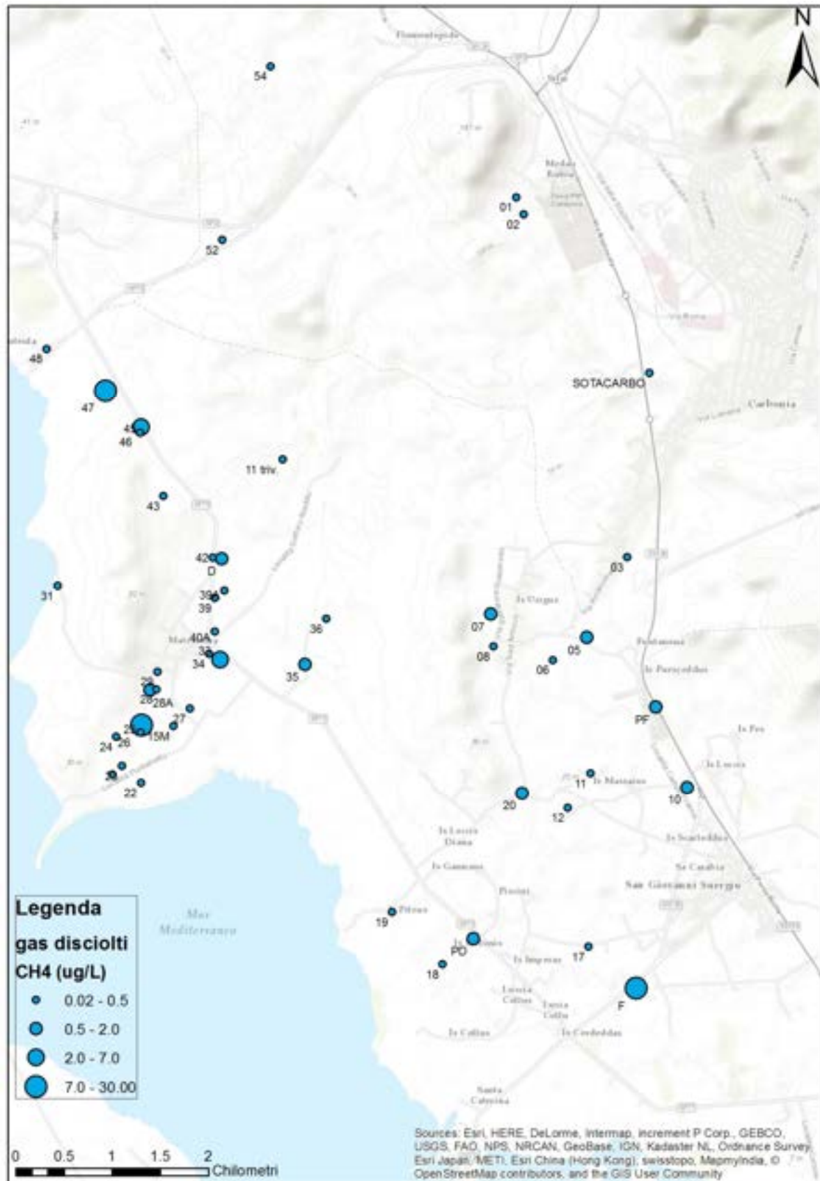
Figura 10. Bubble map che mostra la distribuzione spaziale della concentrazione di CH 4 disciolto.
