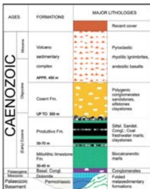
Figura 1. Stratigrafia del Bacino carbonifero del Sulcis (Rossi et al., 2009).
