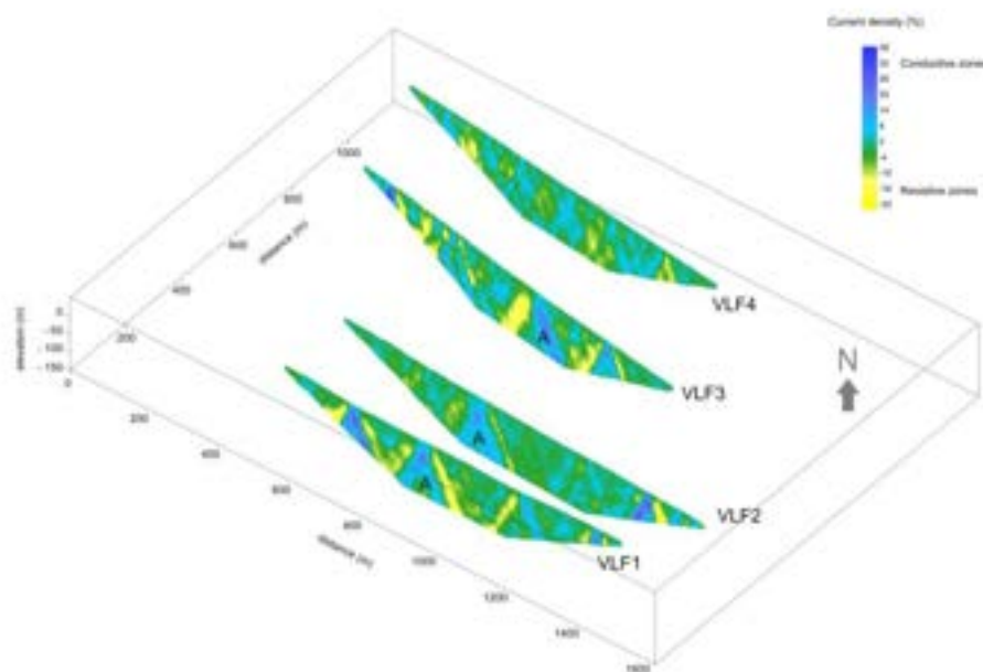
Fig.1 - Visualizzazione 3D delle pseudosezioni di densità di corrente.
