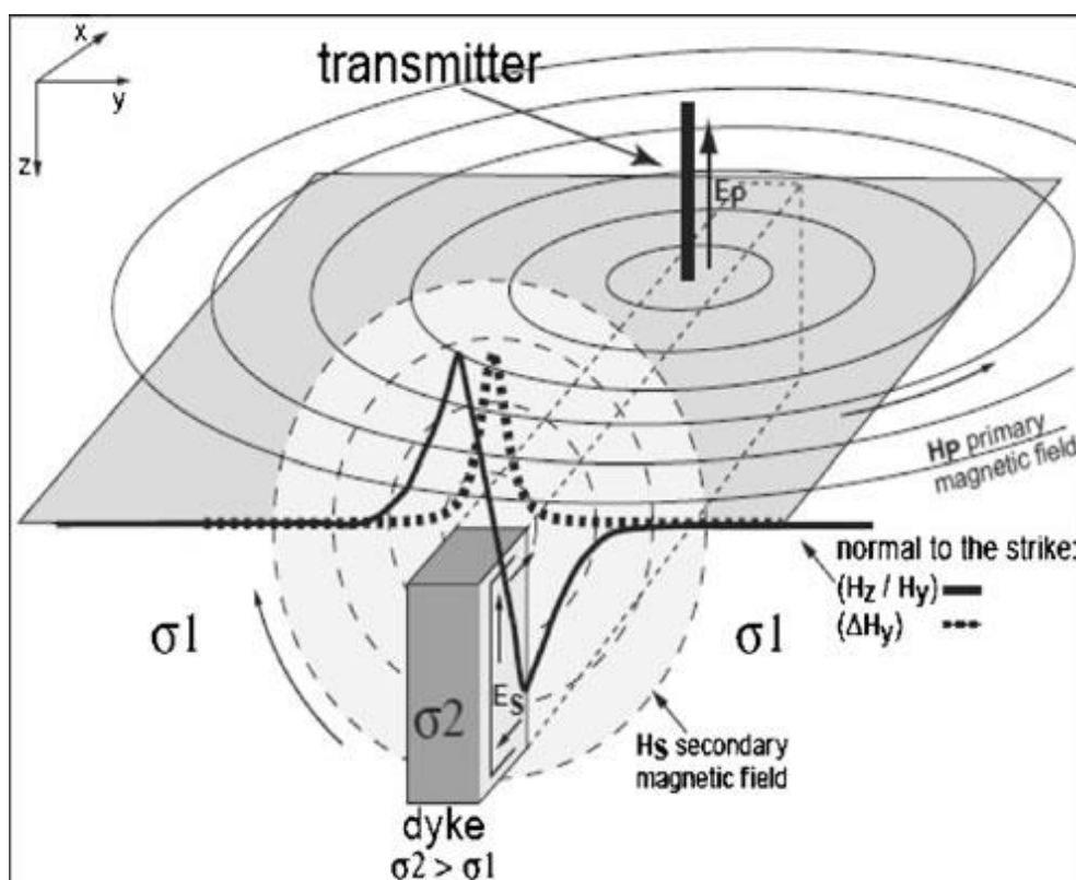
Fig.2 - Distribuzione del campo e.m. nel metodo VLF, in corrispondenza di un corpo conduttore in giacitura verticale. Courtesy from: Bosch and Müller, 2001.
