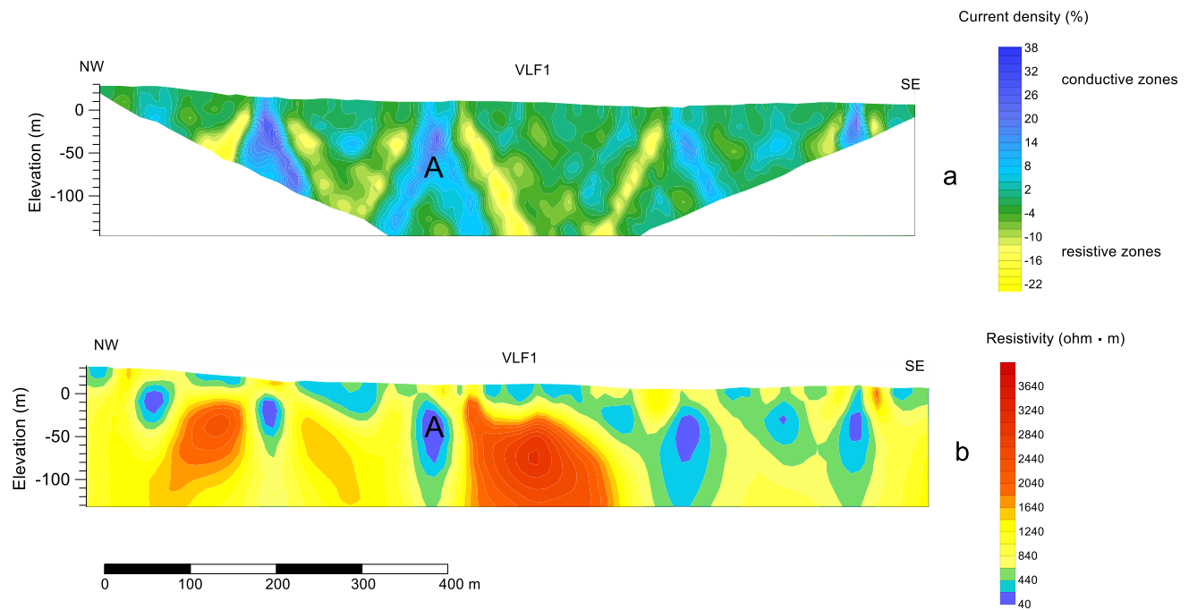
Fig. 9 - Pseudosezione di densita' di corrente (a) e sezione di resistivita' (b), ottenuta mediante l'inversione dei dati, per il profilo VLF1.
