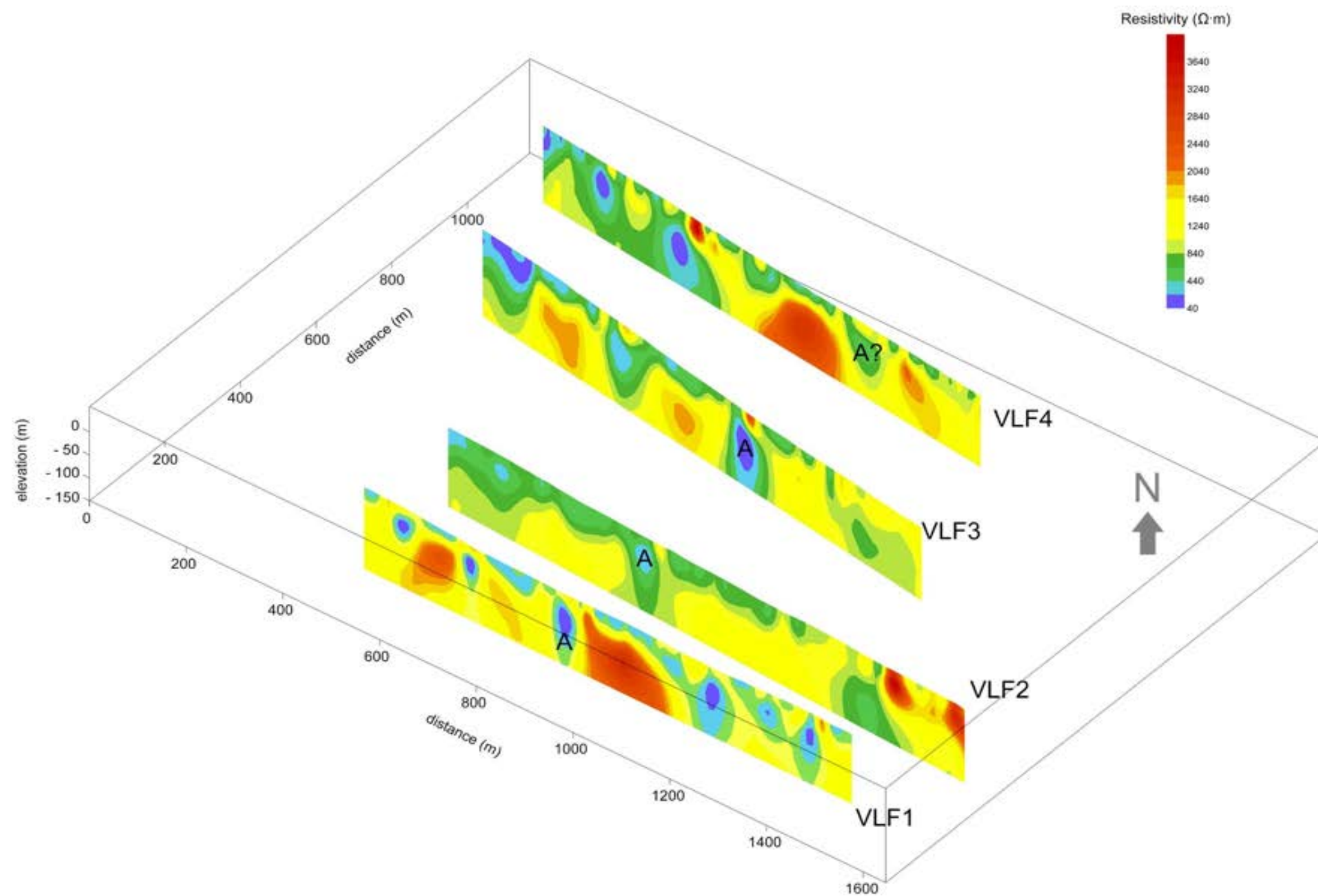
Fig.10 - Visualizzazione 3D delle sezioni di Fig resistività ottenute mediante inversione bidimensionale dei dati VLF relativi ai profili VLF1-VLF4. Fig.10 - 3D Visualization of the resistivity cross-sections obtained by 2D inversion of the VLF data for the VLF1-VLF4 profiles.
