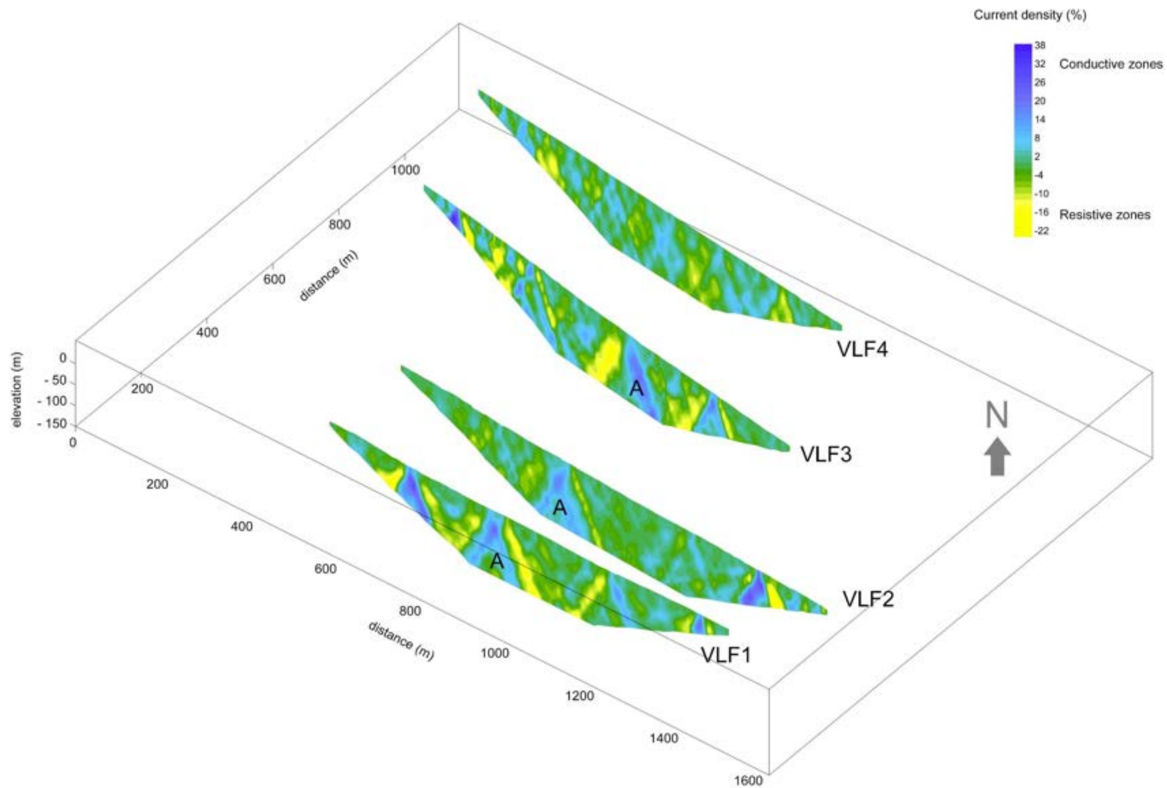
Fig.7 - Visualizzazione 3D delle pseudosezioni di densità di corrente ottenute applicando il filtro Karous-Hjelt ai valori della componente in fase preliminarmente filtrati.
