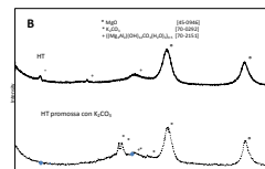
XRD idrotalcite impregnata e non con K 2 CO 3
