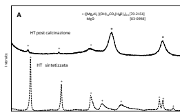
XRD dell'idrotalcite sintetizzata prima e dopo la calcinazione
