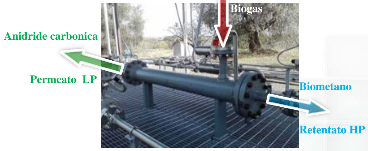
Modulo di upgrading
