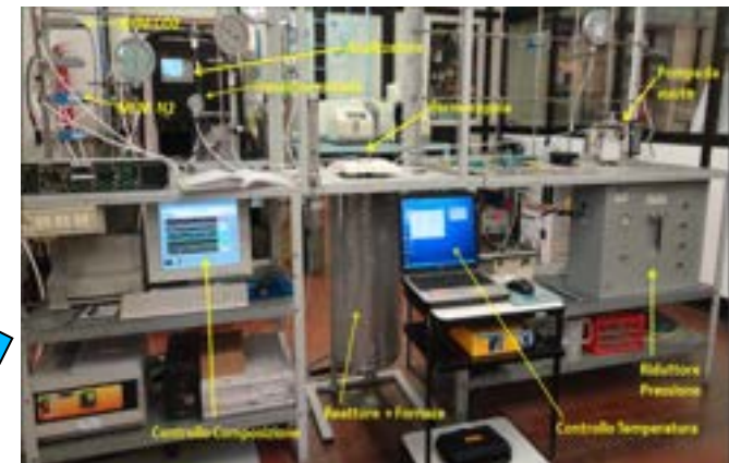
Impianto per la cattura della CO 2
