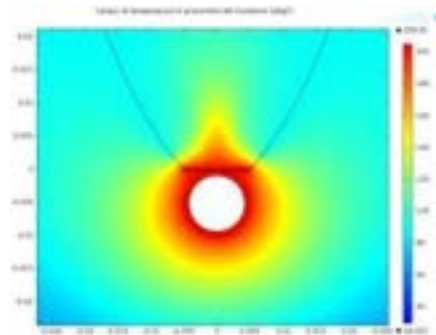
Risultati delle analisi termo-fluidodinamiche effettuate sul modello di concentratore considerato
