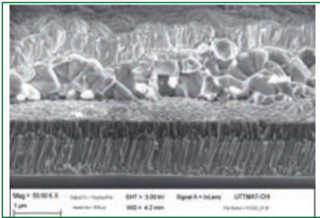
Immagini SEM della sezione di due celle in CZTS fabbricate da precursori ottenuti in condizioni
