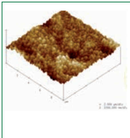
Immagini AFM di \text{ZnO}:\text{B} depositato per LPCVD su vetro testurizzato mediante tecnica Aluminum Induced Texture (sinistra) e di un substrato di vetro nanostrutturato opportunamente progettato (destra)
