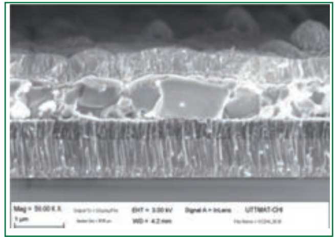
Immagini SEM della sezione di due celle in CZTS fabbricate da precursori ottenuti in condizioni
