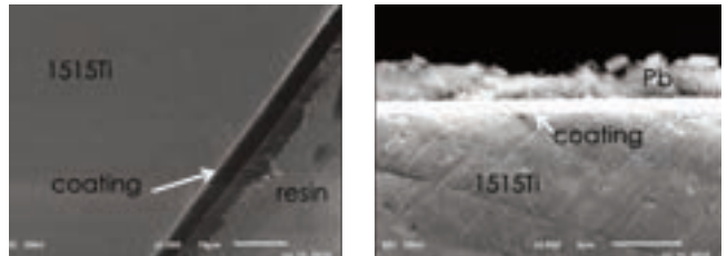
Foto al SEM di campioni ricoperti di allumina (senza buffer intermedio) mediante tecnica "Pulsed Laser Deposition" (IIT@POLIMI), esposti in piombo ad elevata temperatura. Non sono presenti fenomeni corrosivi
