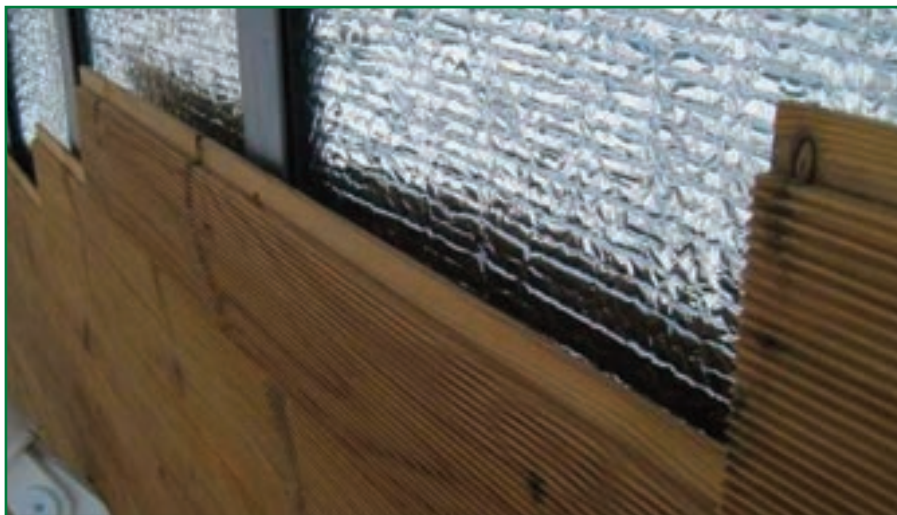
Esempio di cappotto esterno riflettente (SA.M.E.): strato esterno in ossido di magnesio; Isoliving in doppio strato; montanti a pettine in ABS (studiati in modo tale da assicurare la posa corretta dell'isolante riflettente)
